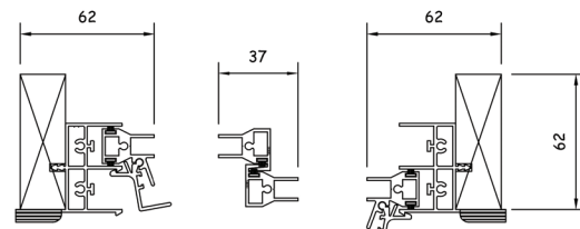
Jamb Detail
